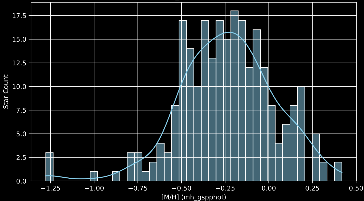
GALAH DR4 Field: [7140] [M/H] (mh_gspphot) (n= 252)
