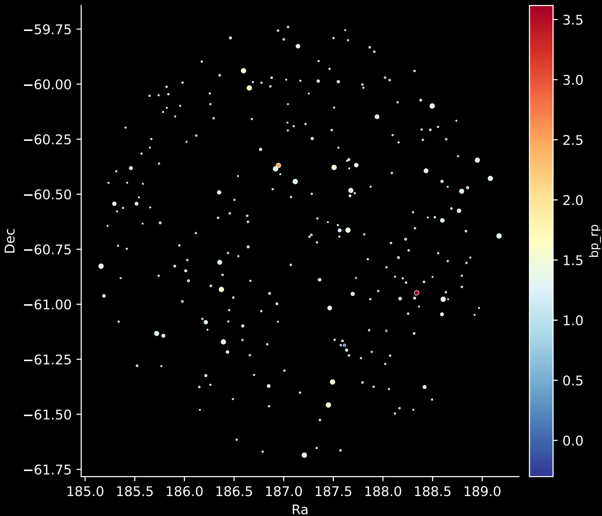
GALAH DR4 Field: [7140] Stars: 253
