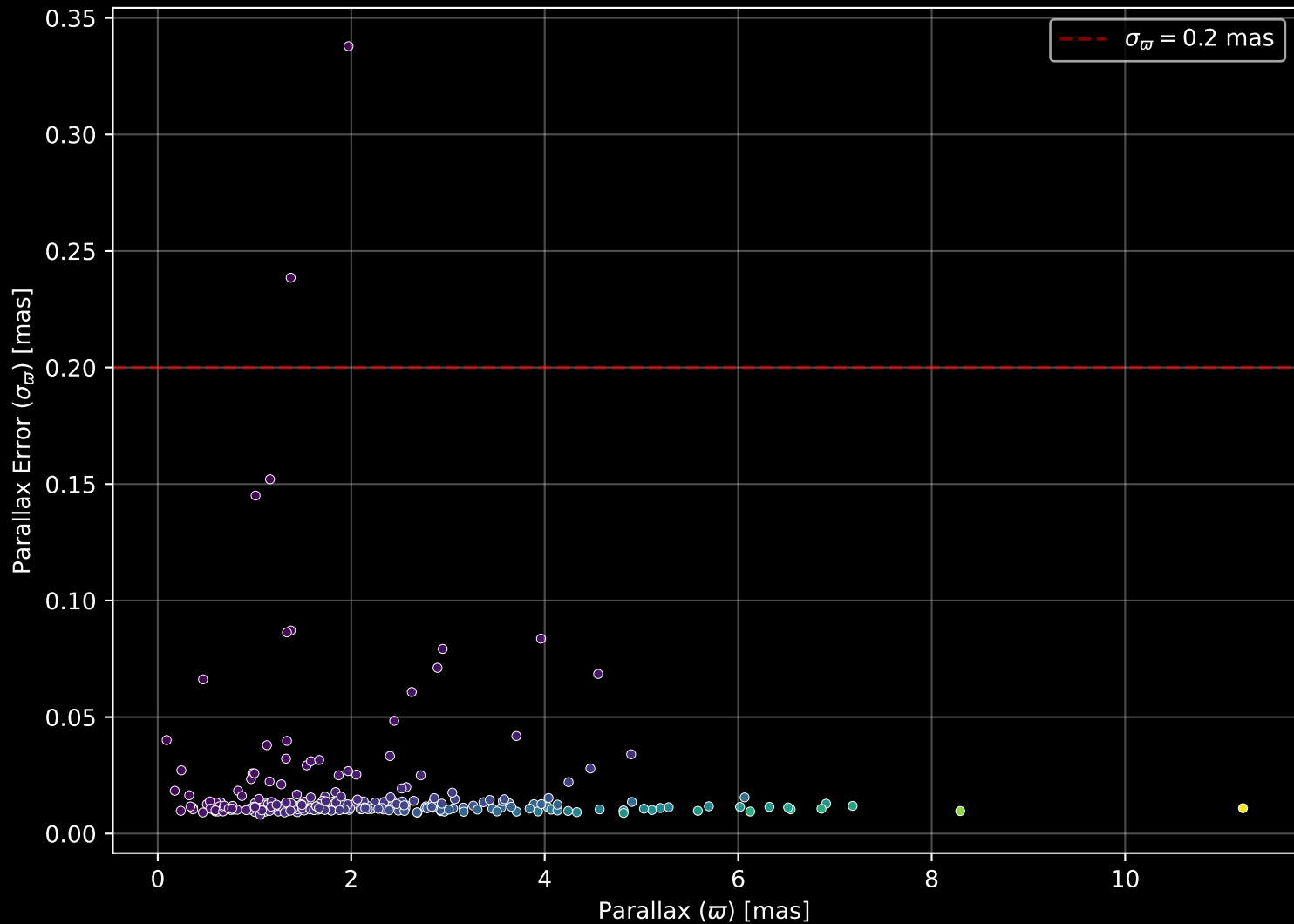
GALAH DR4 Field: [7140] Parallax Quality (n= 253)
