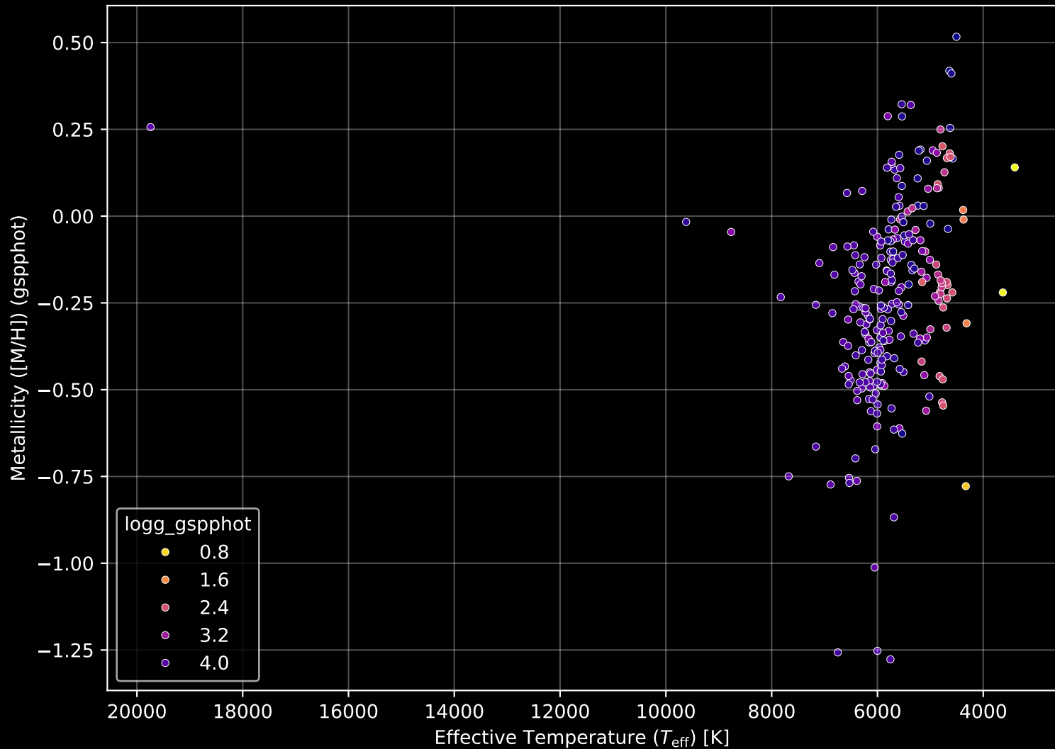
GALAH DR4 Field: [7140] Stellar Population Parameters (n= 253)
